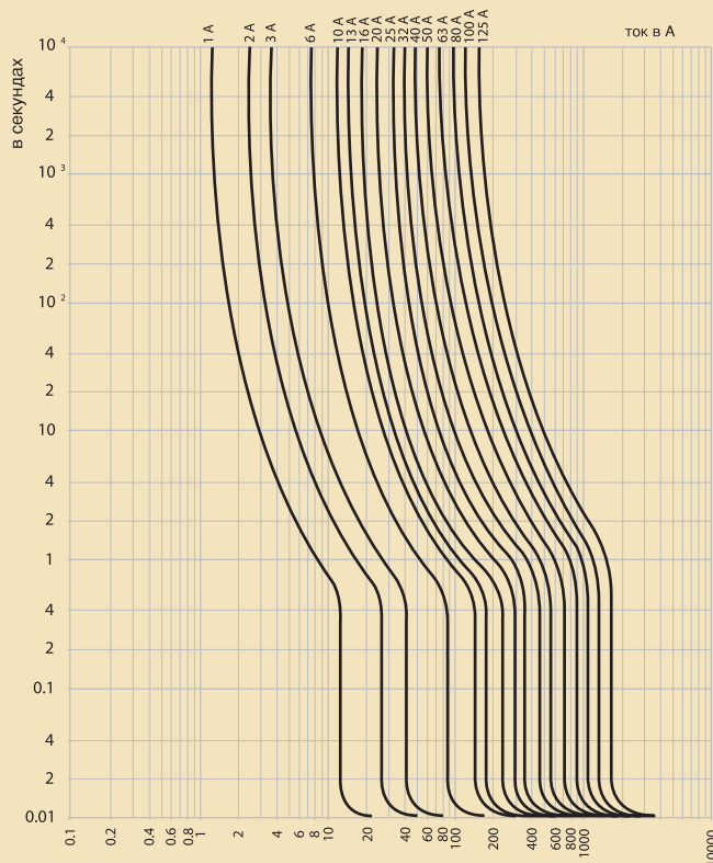
Соответствуют МЭК 60898, Тип D, уставка защиты от КЗ 10 - 20 In
